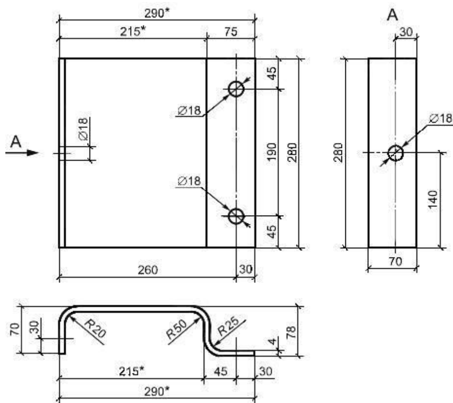
Рисунок 11 - Консоль-амортизатор КА
