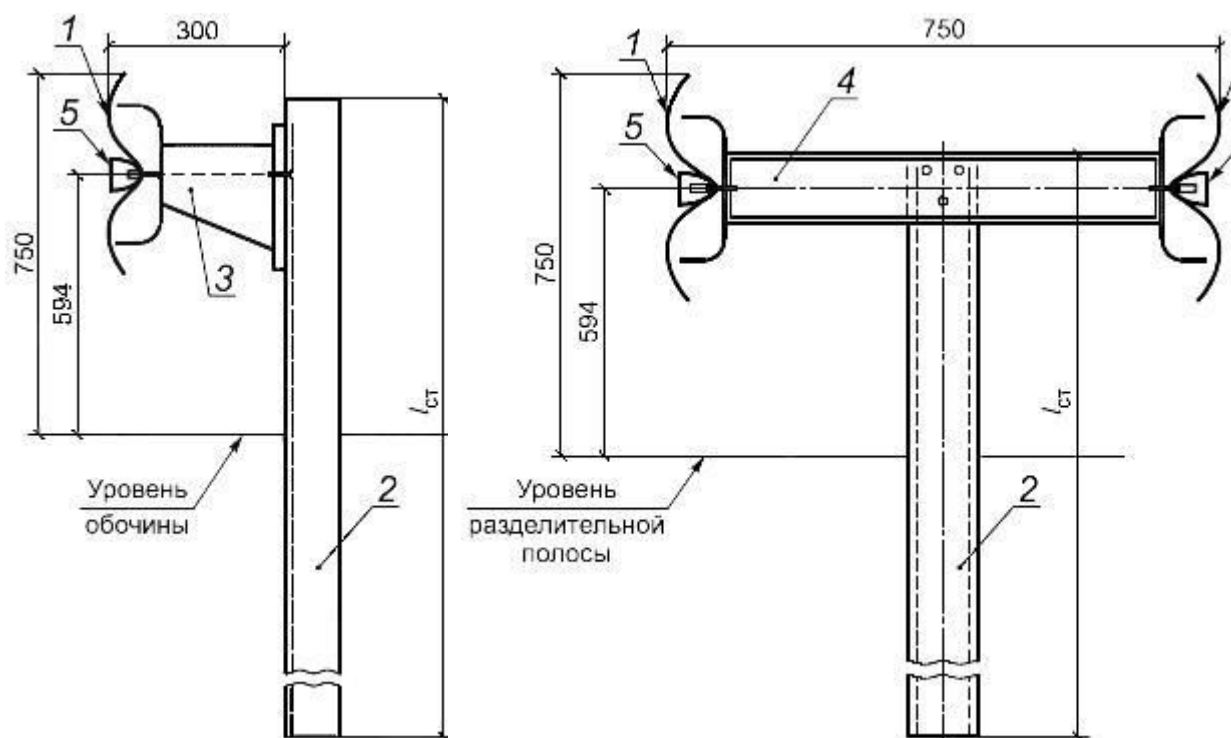
а) Одностороннее ограждение
