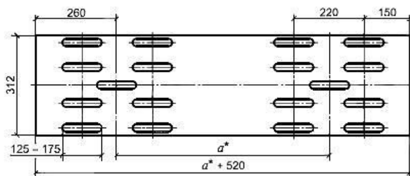
Рисунок 6 - Секция балки-вставки СБВ над деформационным швом
