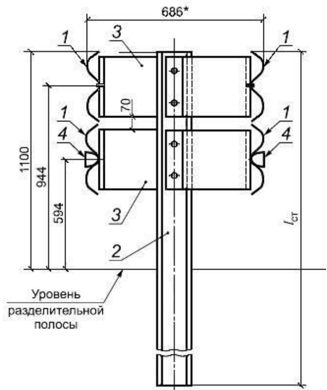
г) Двухстороннее двухъярусное ограждение
