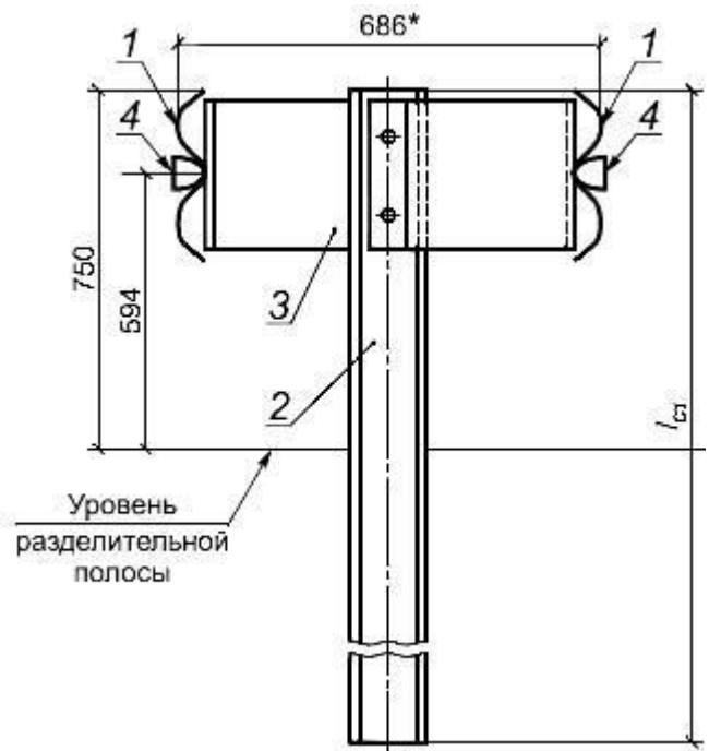
б) Двухстороннее одноярусное ограждение
