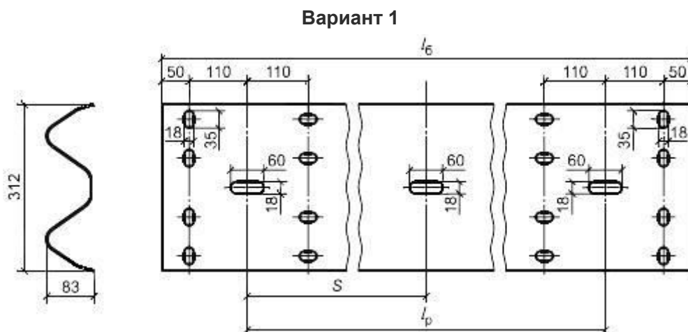
Рисунок 4 - Секция балки ограждений СБ
